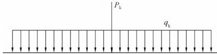
图 B.0.1-1 车道荷载
