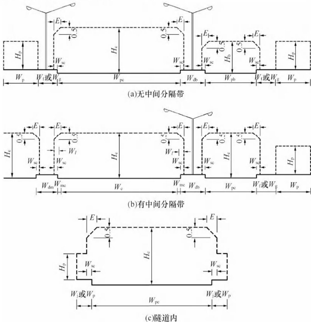
图 A.0.1 道路建筑限界
